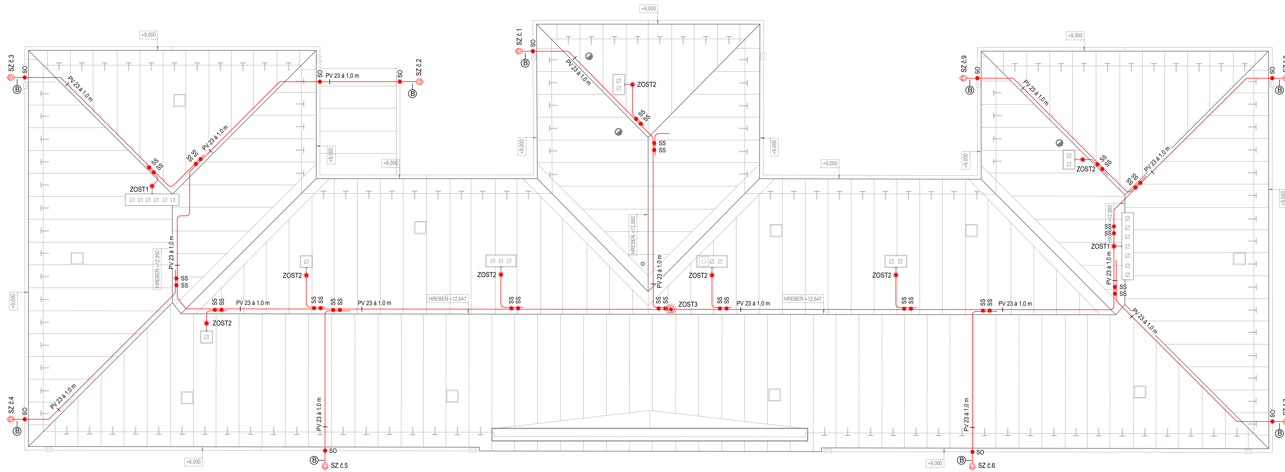
PÓDORYS STRECHY/ M 1:75
